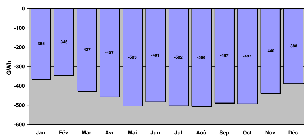
Bilan énergétique - Scénario revente - Année 2010
