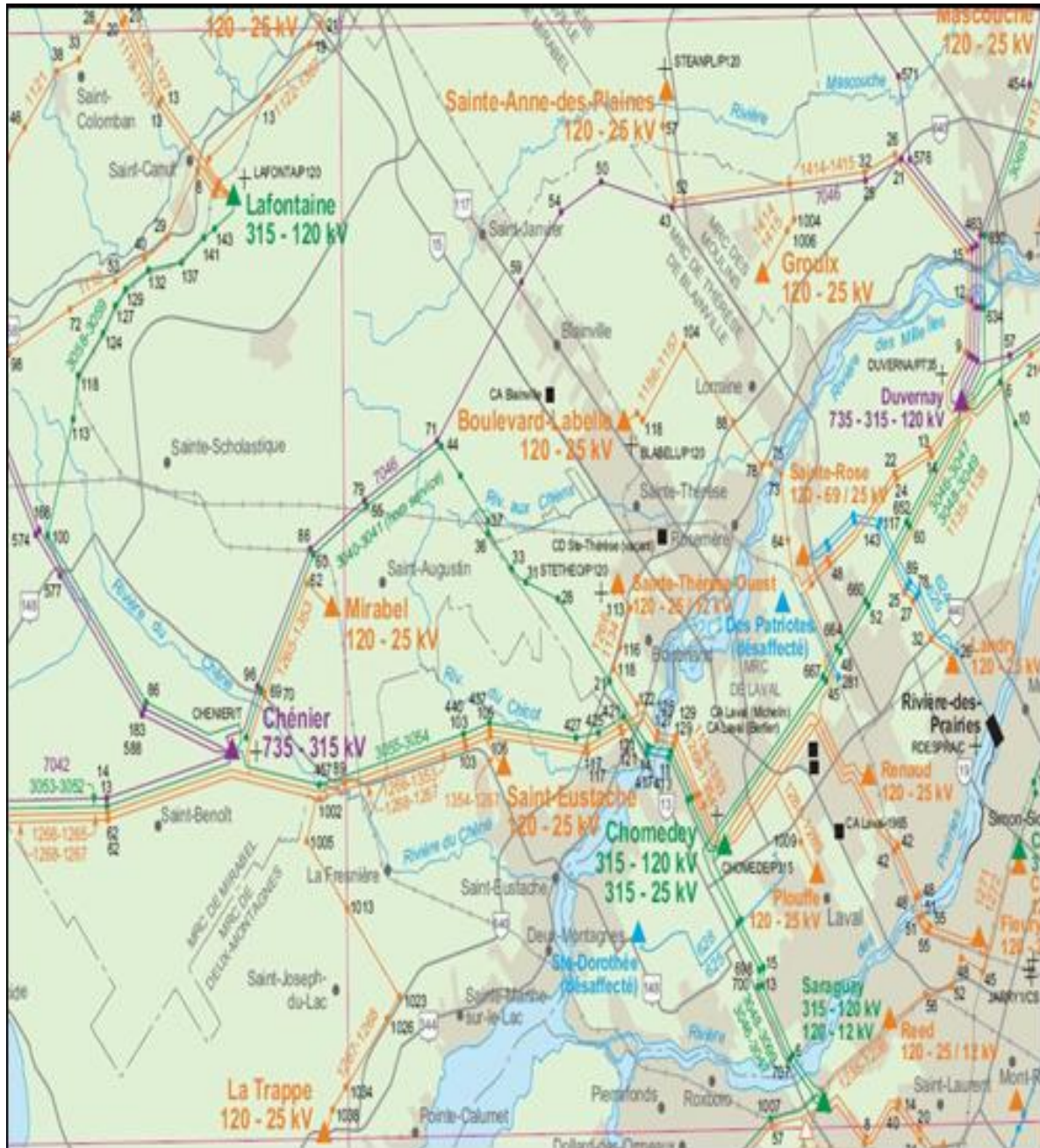
Figure 1 Emplacement des postes du réseau de transport régional dans la zone d'étude
