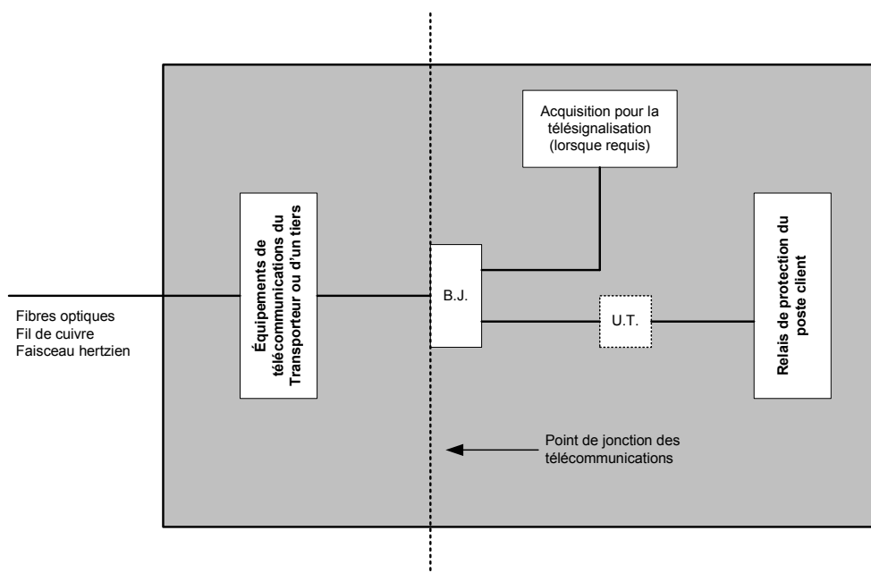
Figure 2 Système de télécommunications du poste client
