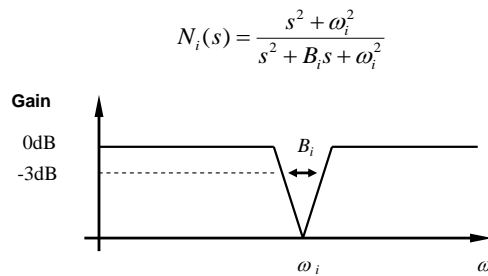
Figure 3 – Caractéristiques des filtres coupe-bande
