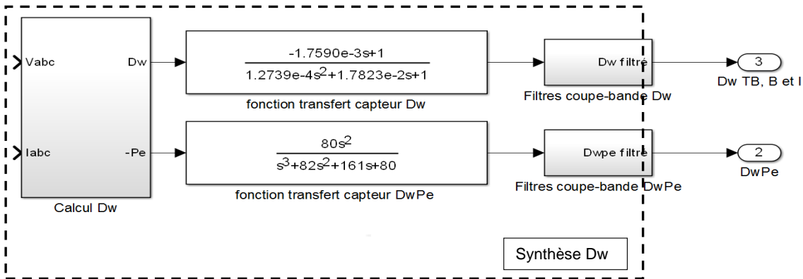
Figure 2 – Synthèse de la vitesse du rotor
