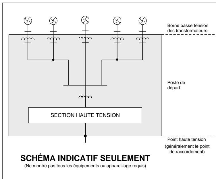
Figure 5 – Poste de départ d'une centrale éolienne
