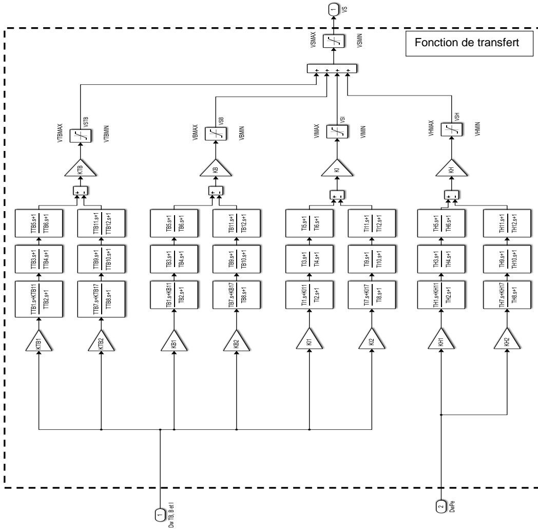
Figure 4 – Fonction de transfert du stabilisateur multibande
