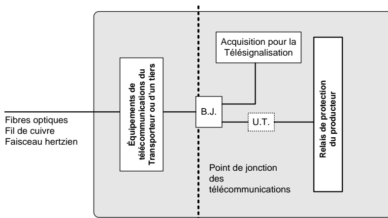
SCHÉMA DE PRINCIPE SEULEMENT
