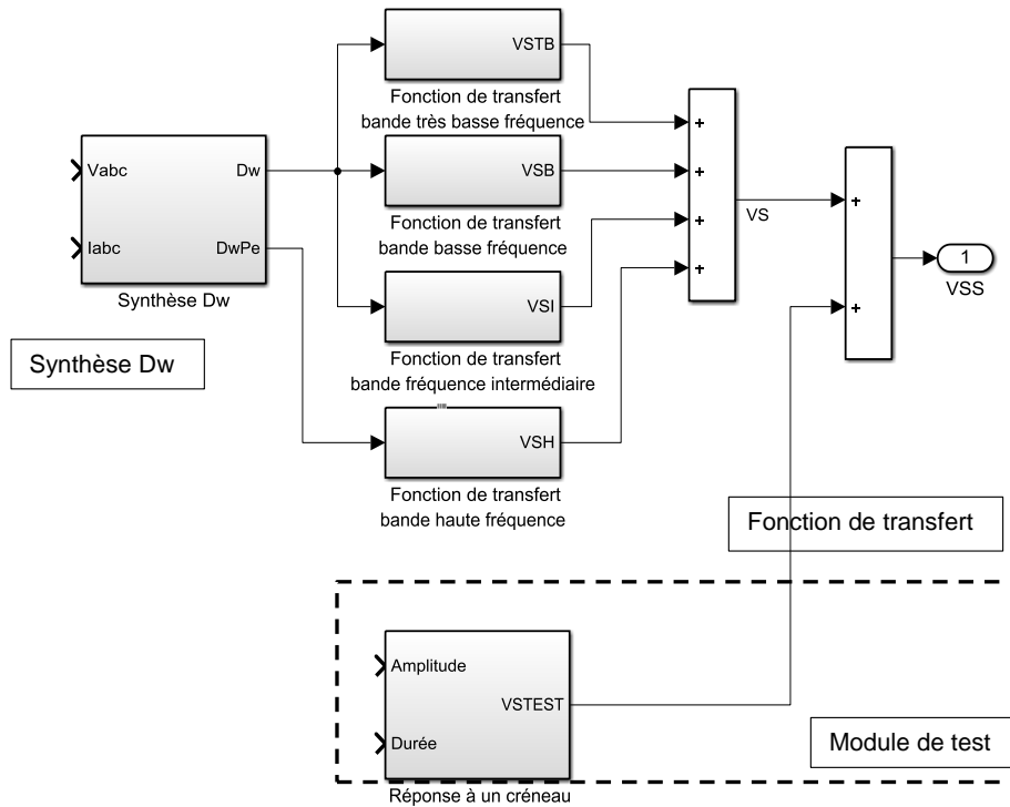
Figure 1 – Schéma simplifié du stabilisateur multibande
