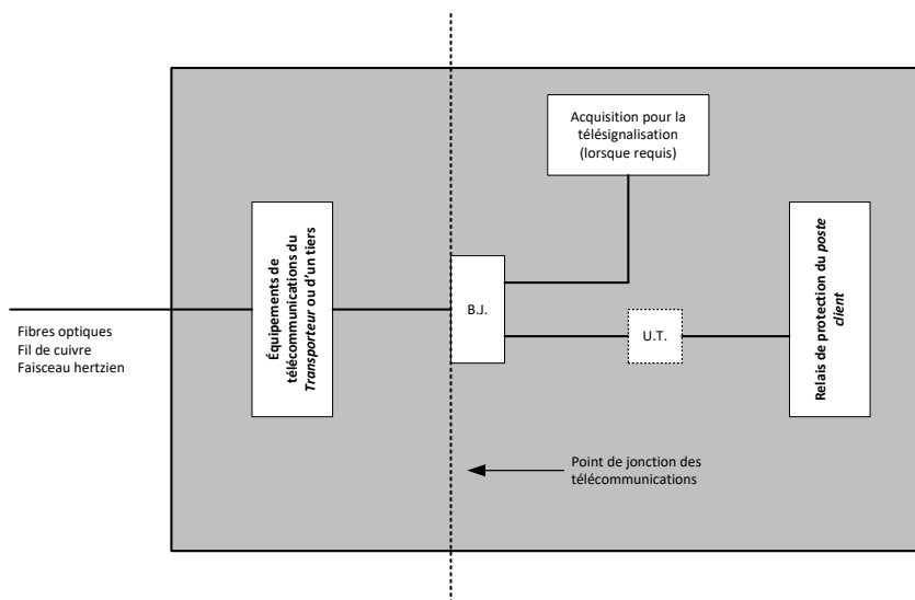
Figure 2 Système de télécommunications du poste client
