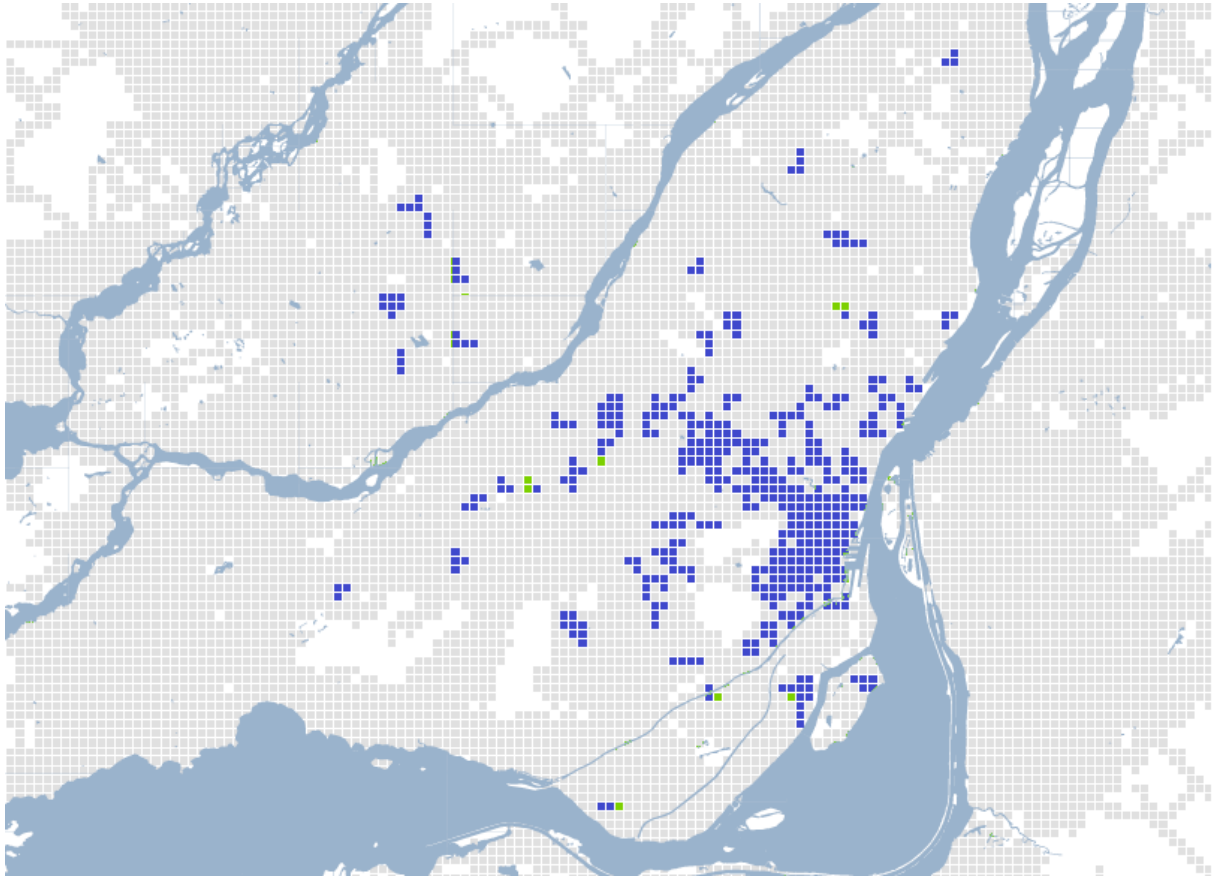
FIGURE E-1.2 : CRITÈRE DE DEM D'AU MOINS 50 MVA PAR KM 2 SUR UNE DISTANCE MINIMALE DE 2 KM DE RÉSEAU
