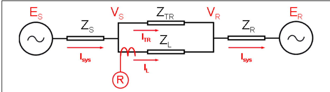
Figure 3 : Impédances du réseau vues par le relais R (les raccordements de tension ne sont pas illustrés).
