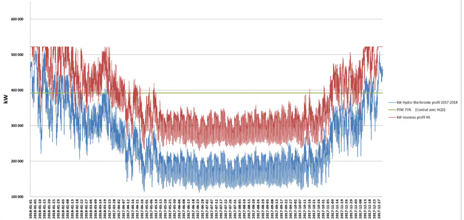
kW Hydro-Sherbrooke profil 2017-2018
