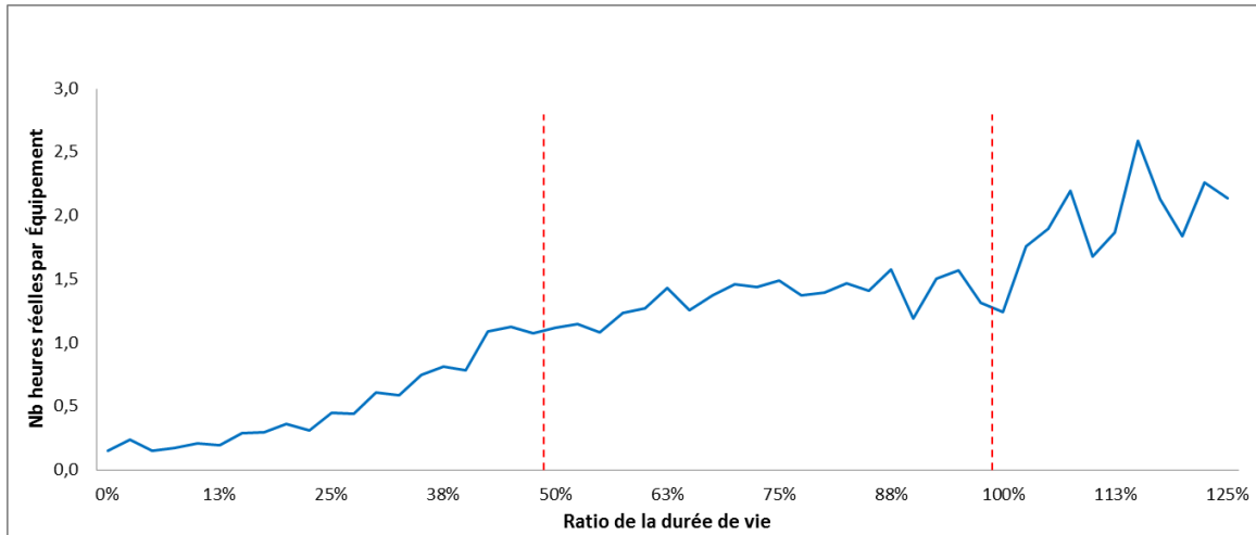
Figure 1 Hausse des heures de maintenance requises en fonction de la durée de vie
