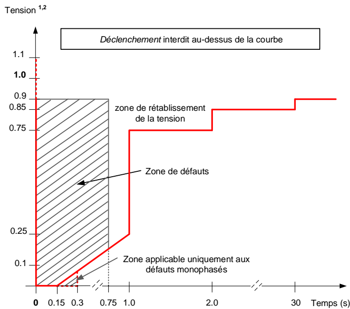
Figure 6 : Sous-tension durant laquelle la centrale utilisant des SERMQ doit demeurer en service (Low Voltage Ride Through) à la suite d'une perturbation
