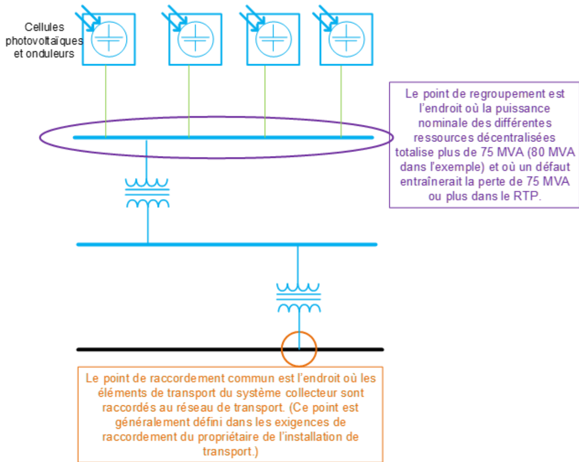
Figure I4-16 : Exemple d'une centrale photovoltaïque comportant plusieurs niveaux de transformation de tension
