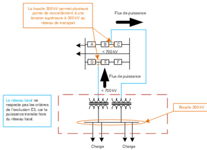
Figure E3-35 : Réseau local avec boucle à 300 kV
