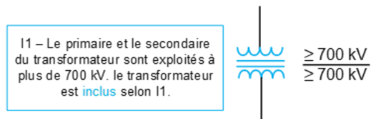
Figure I1-1 : Transformateur typique exploité à plus de 700 kV
