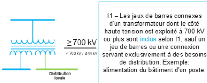
Figure I1-4 : Transformateur dont le primaire est exploité à plus de 700 kV et ligne servant à des besoins de distribution
