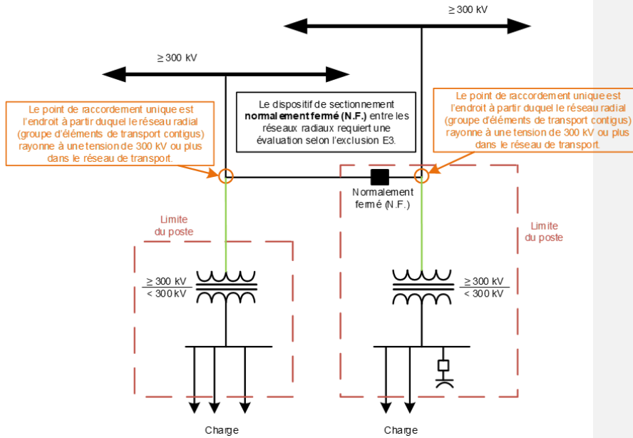
Figure E1-29 : Dispositif de sectionnement normalement fermé entre deux réseaux radiaux alimentant des charges
