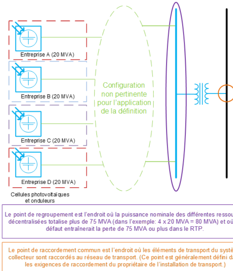
Figure I4-17 : Exemple d'une centrale photovoltaïque dont les installations de production appartiennent à différents propriétaires
