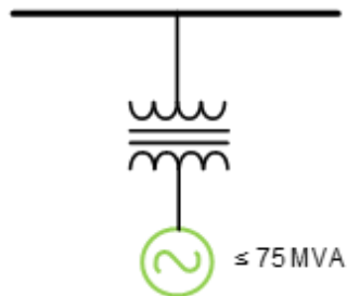
Figure I2-8 : Ressource de production de 75 MVA ou moins
