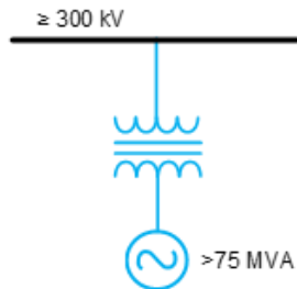
Figure I2-6 : Ressource de production de plus de 75 MVA raccordée au RTP
