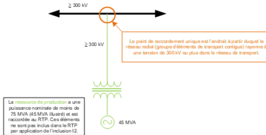
Figure E1-31 : Réseau radial comportant une ressource de production, exclu du RTP
