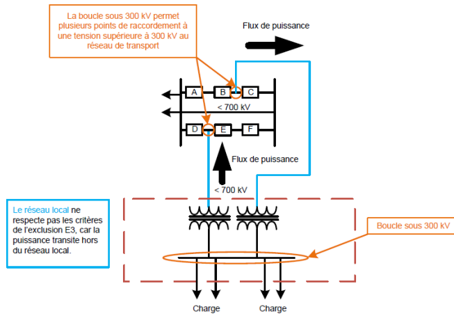
Figure E3-35 : Réseau local avec boucle à sous 300 kV
