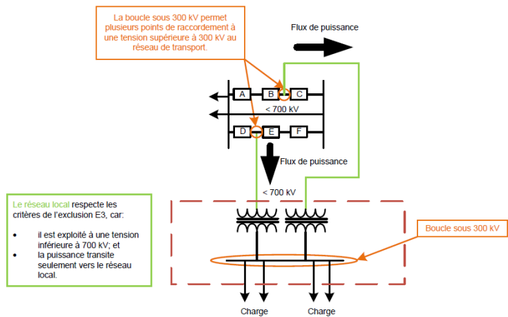
Figure E3-34 : Réseau local avec boucle sous à 300 kV
