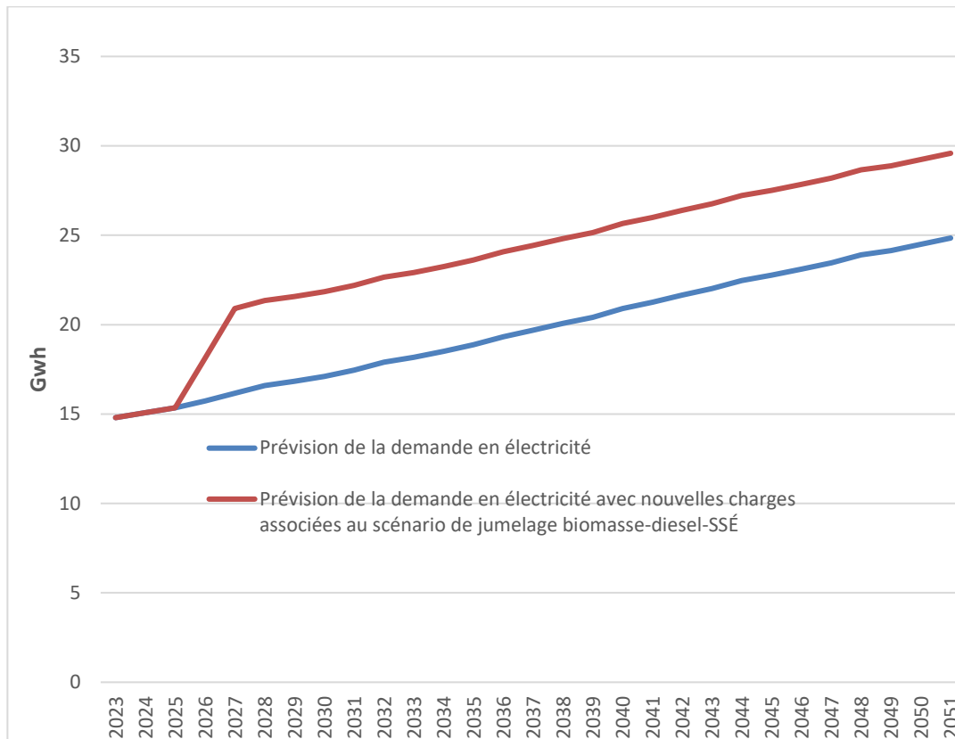
FIGURE 4 RÉVISÉE : PRÉVISION DES BESOINS EN ÉNERGIE À OPITCIWAN SUR LA DURÉE DU CONTRAT
