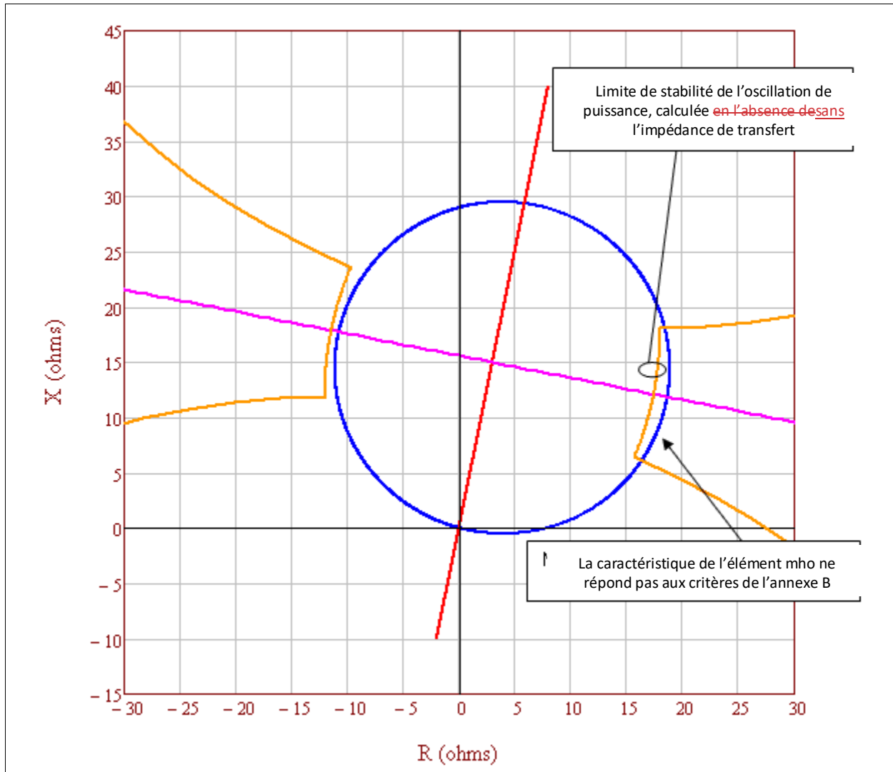
Figure 10 : Exemple de région d'oscillation de puissance instable (tracés orange) en l'absence de sans l'impédance de transfert parallèle. La caractéristique de l'élément mho du relais (cercle bleu) ne répond pas au critère A de l'annexe B de la norme PRC-026-12, car elle n'est pas entièrement circonscrite par la région d'oscillation de puissance instable.
