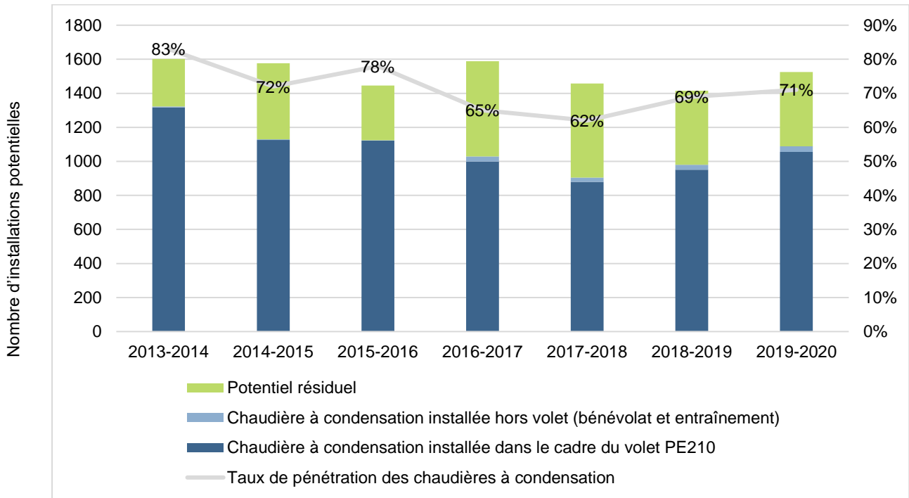
Figure 1 : Taux de pénétration des chaudières à condensation
