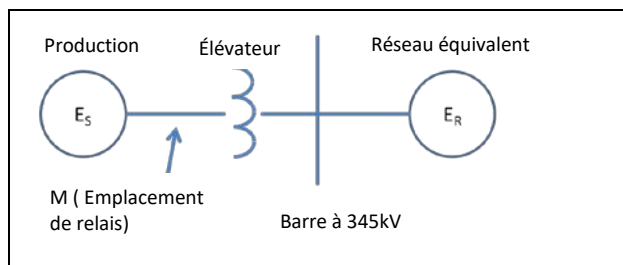
Figure 17 : Schéma unifilaire simplifié du réseau à évaluer.
